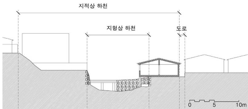
손가정 노인정과 정릉천 지역 실측단면도(©생활건축연구소)
